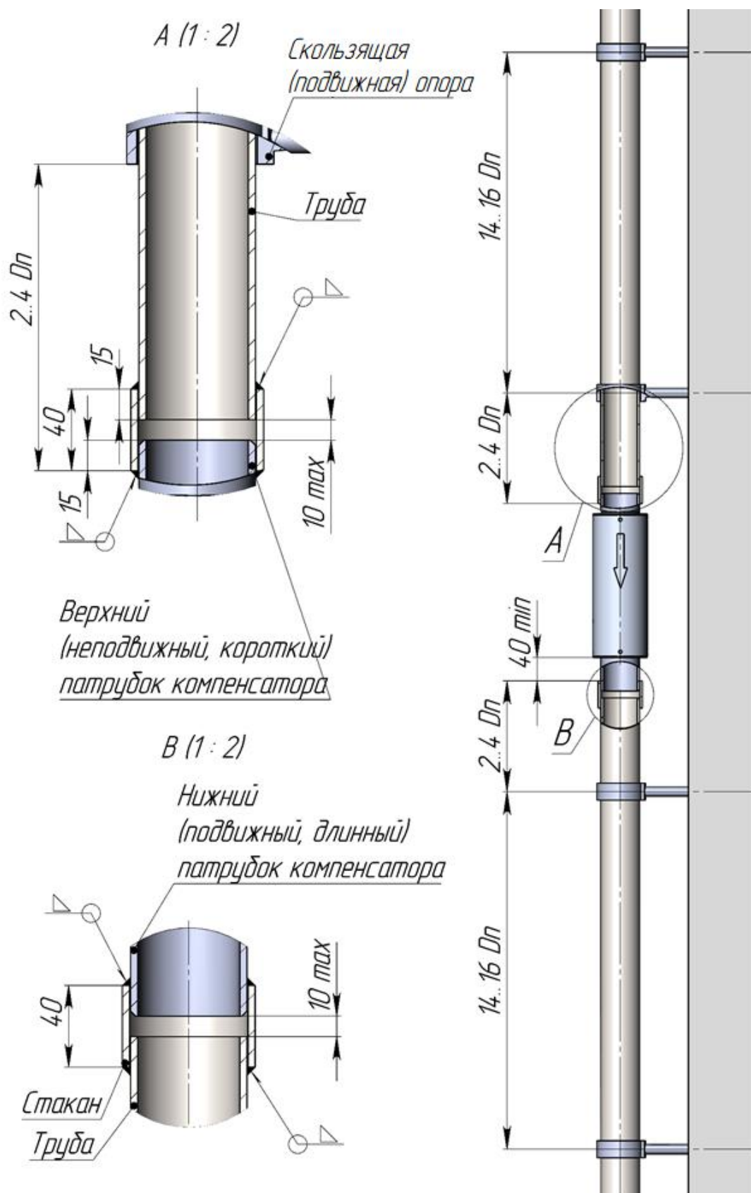
Рис. 18.1 Схема установки компенсатора на трубе D_n < 25 \text{ мм} через приварной стакан (муфту)
