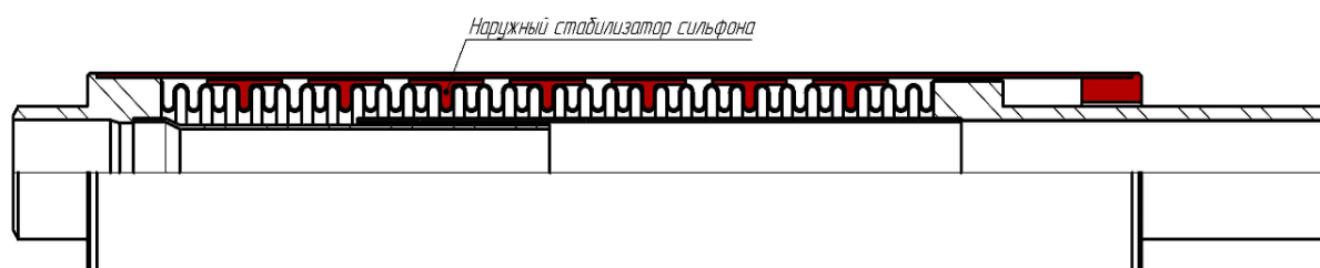
Рис. 8.1. Схема сифонного компенсатора с наружным стабилизатором сифона
