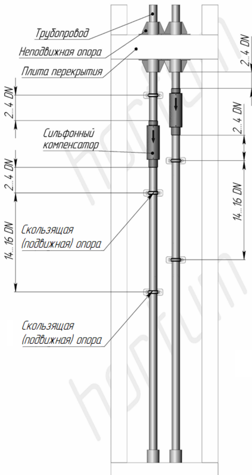
Схема 15. Установка в узких шахтах неподвижных опор и компенсаторов
