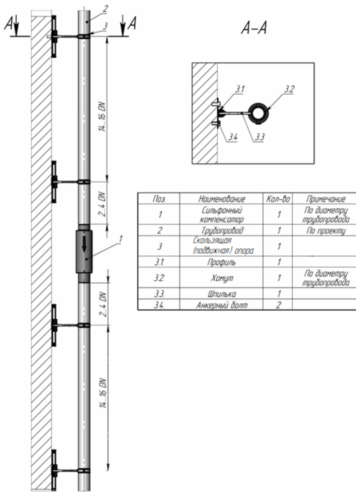
Схема 14. Установка подвижных (скользящих) опор
